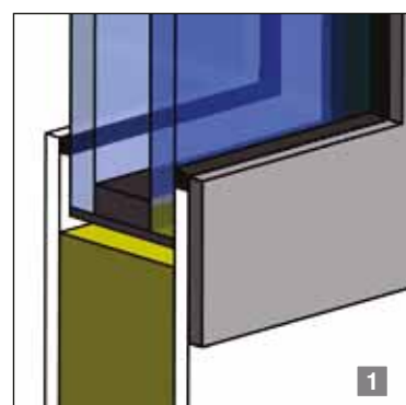
Basic Line 1. außen aufgesetzter Edelstahlrahmen, innen rahmenlos. Standard Basic-Line.
